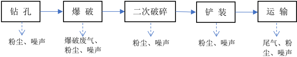
图 2-1 整体生产工艺流程
