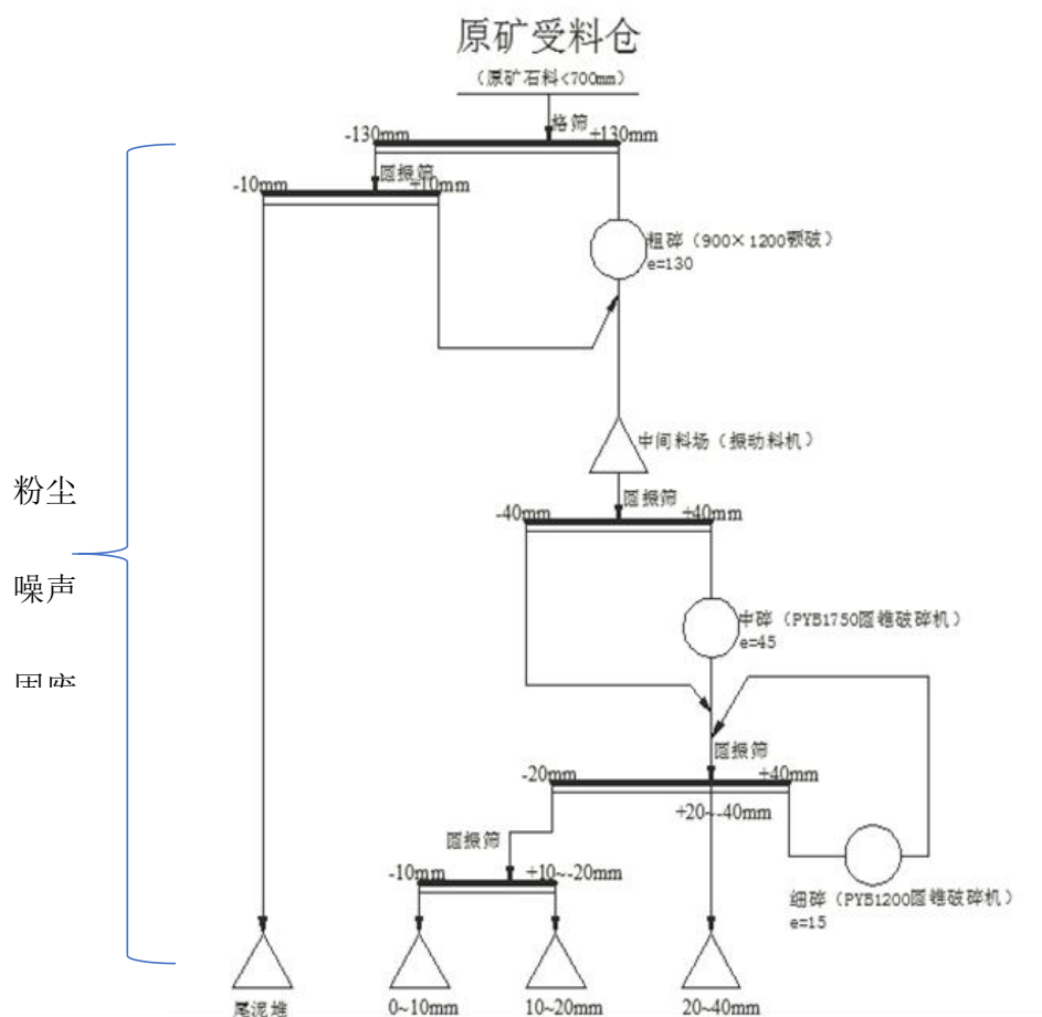
图 2-2 破碎筛分生产工艺流程图
