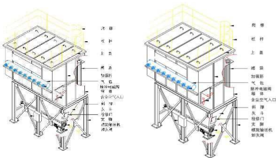
图 6.2-2 脉冲布袋除尘器结构图
