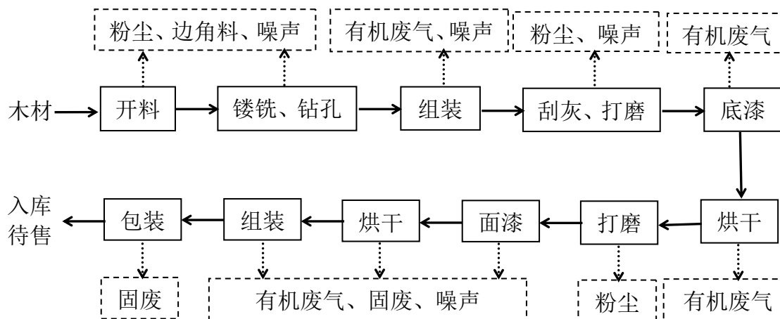
图3 家具生产工艺及产污节点示意图
