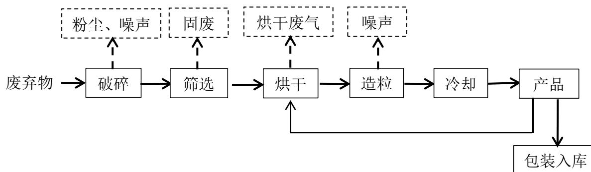
图3 RDF燃料颗粒产污节点图
